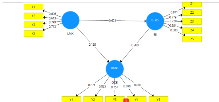
Gambar 1 Hasil Pengujian Diagram Jalur Model Pengukuran PLS (Outer Model)
