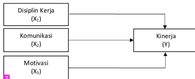
Gambar 1. Kerangka Konseptual
