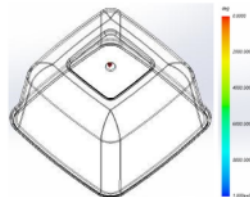
Gambar 11. Hasil Analisa Cacat Produk Weldlines
