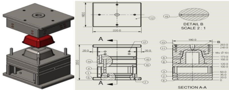
Gambar 13. Hasil Pembuatan 3D Modeling Molding
