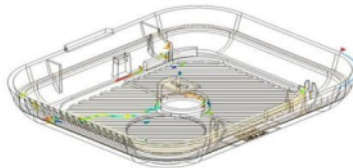
Gambar 6. Kondisi Produk Weldlines
