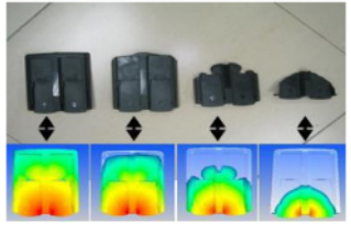
Gambar 3. Kondisi Produk ShortShot
