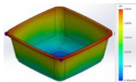
Gambar 12. Hasil Analisa Cacat Produk Air Trap
