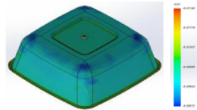
Gambar 10. Hasil Analisa Cacat Produk Sinkmark
