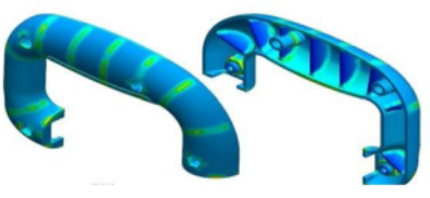
Gambar 4. Kondisi Produk Sinkmark
